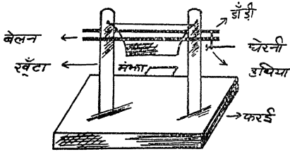
लंगोटा चरखी और उसके अंग ( रेखाचित्र ८८ )
